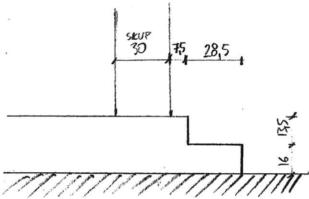
PRZEKROJ A-A
